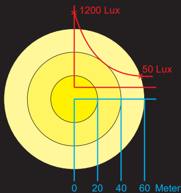
Beispiel 2 Radiales Lichtfeld bei 50° Neigung
