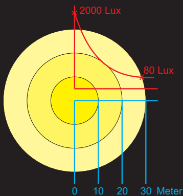
Beispiel 1 Radiales Lichtfeld bei 25° Neigung
